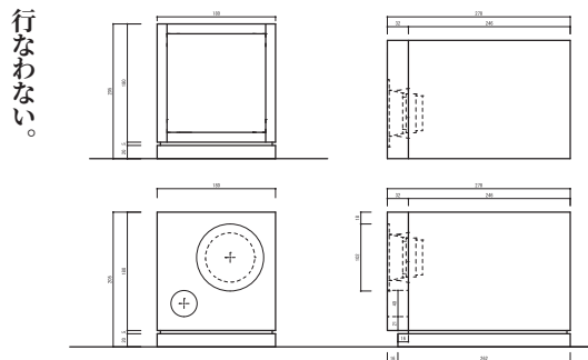
俺流ミニスピーカー構想の図面 立方体のデザインが理想的だが、容積は聴いて調整するため試作機では、後ろを長めに余裕をもって作る
